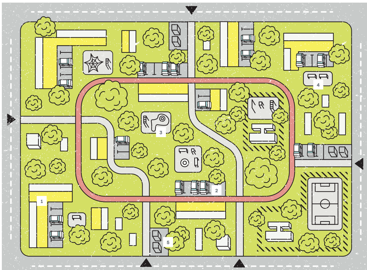
▲ Илл. 16. Принципы размещения функциональных зон при благоустройстве дворов в высокоэтажной микрорайонной застройке
