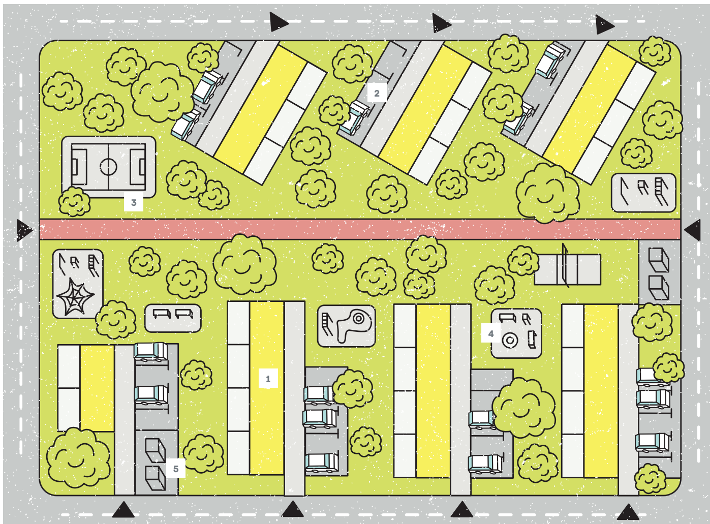
▲ Илл. 14. Принципы размещения функциональных зон при благоустройстве дворов в среднеэтажной микрорайонной застройке
